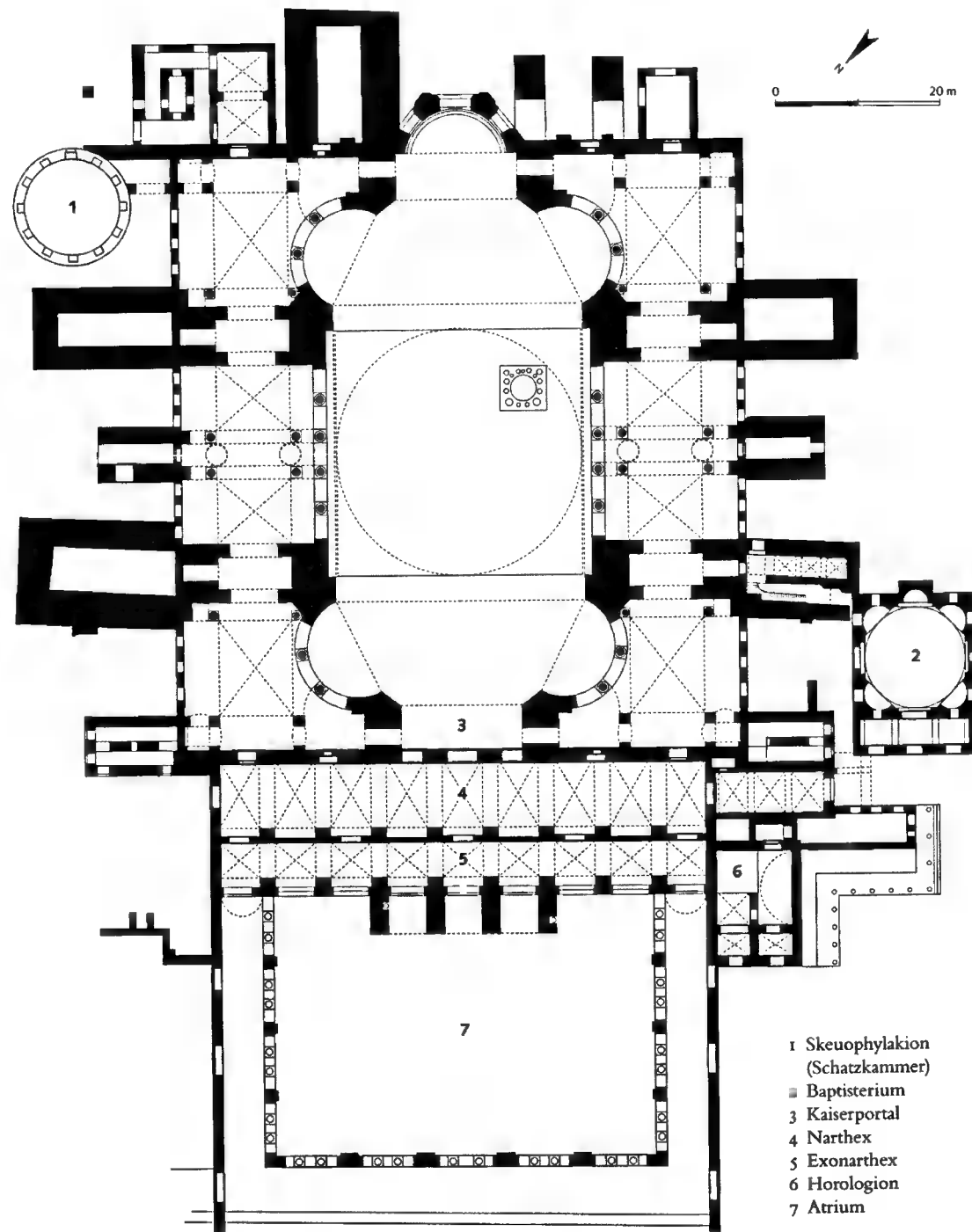
Konstantinopel. Hagia Sophia; 532–537 und 558–563 n. Chr. (Grundriß).
